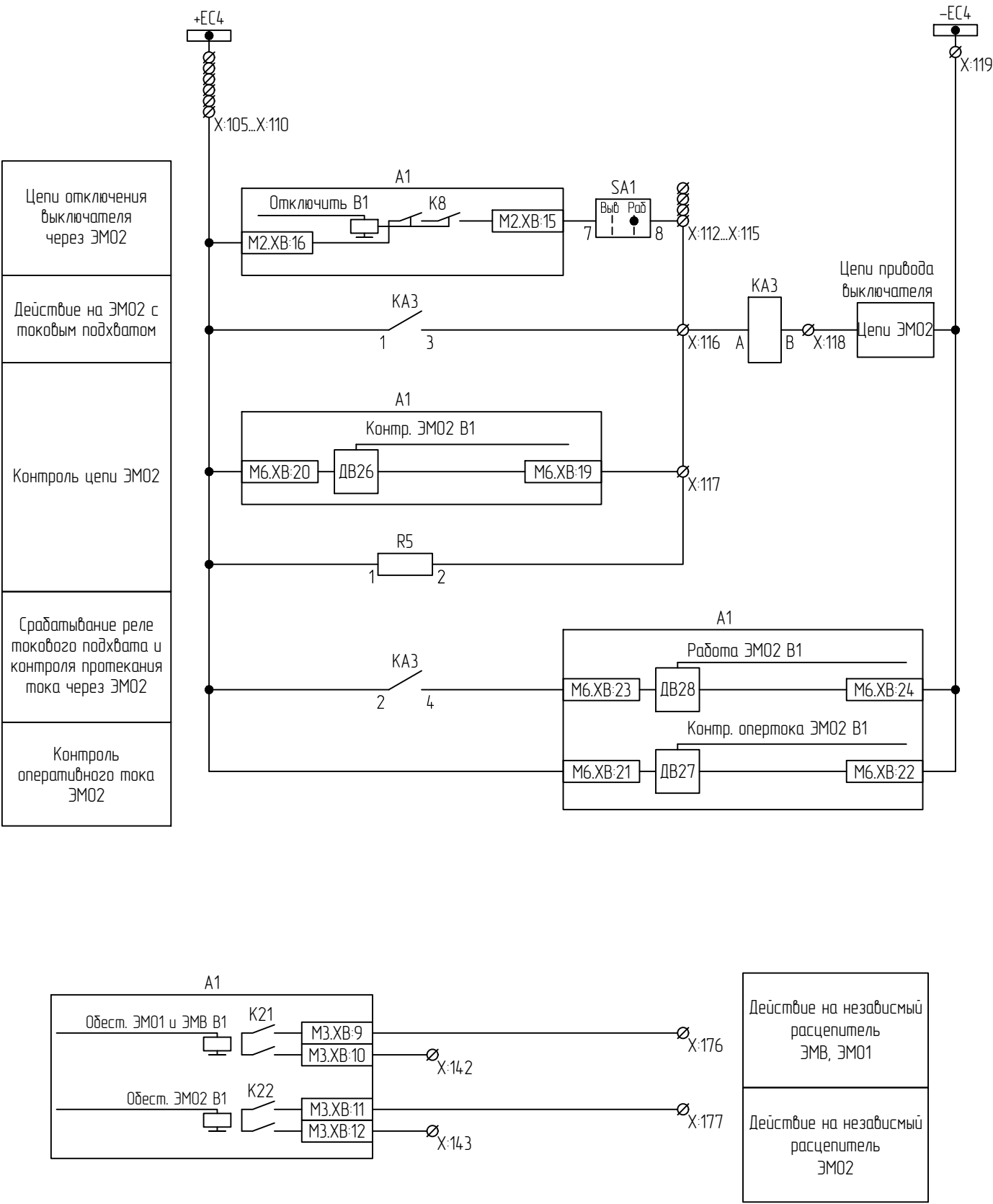
Цепи ЭМ02
